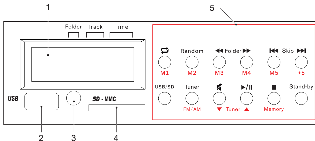
Rysunek 8.3: Moduł źródła sygnału audio
