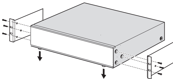
Rysunek 5.1: Montaż jednostki w szafie typu rack 19"
